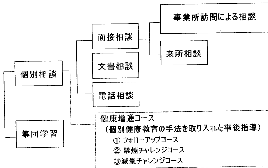
図1: 手法
