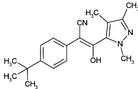
代謝物 BP3
