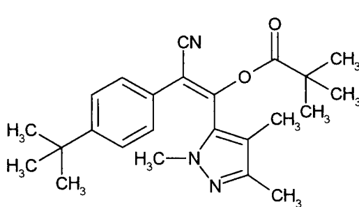
代謝物 BP2
